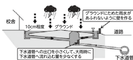
オンサイト貯留施設のイメージ図
