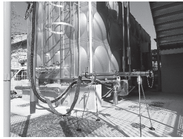
機材をつないだ学校受水槽 (安井小学校)
